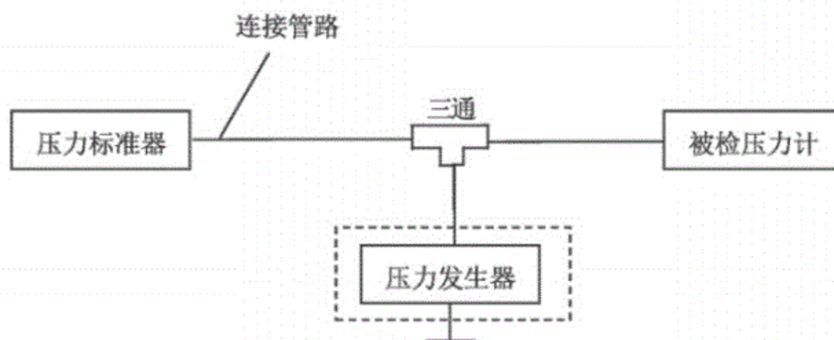
图 2 压力计的示值误差检定连接示意图
