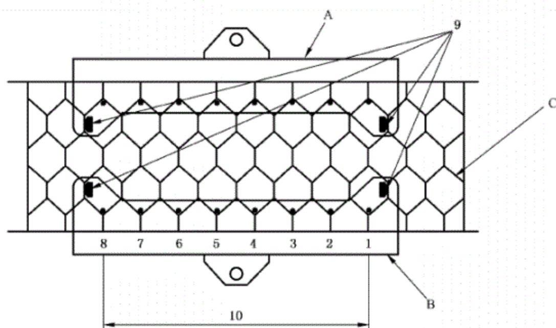
图 A.2 6×8 型钢丝网夹持示例
