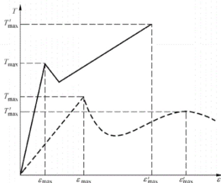
图1 典型负荷-伸长率曲线
