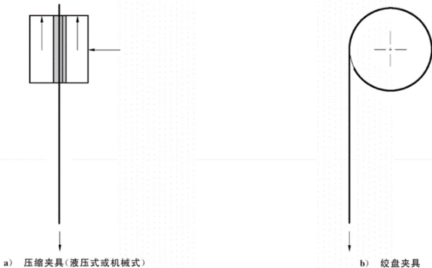
图 3 土工合成材料拉伸试验用钳口面示例
