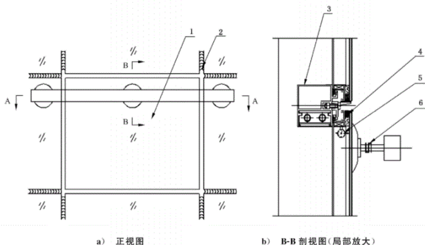
图 1 仪器设备及安装示意图
